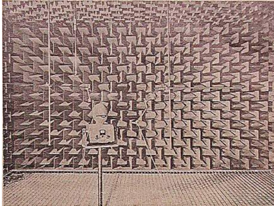
La chambre sourde du laboratoire du Comité consultatif international - télégraphique et téléphonique de l'UIT et une bouche artificielle typique utilisée pour relever la caractéristique de transmission d'un système émetteur téléphonique.
