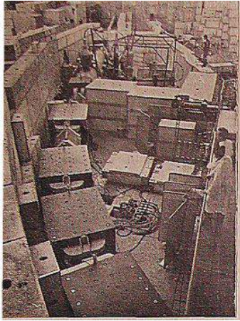
Vue de l'appareillage du transport, de faisceaux dans la salle d'expériences, montrant 4 aimants de déflexion, 2 lentilles quadrupolaires de focalisation ainsi qu'un séparateur électrostatique. (Photo CERN)
